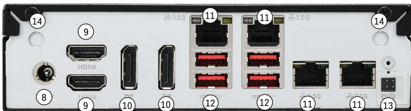
Rückseite
